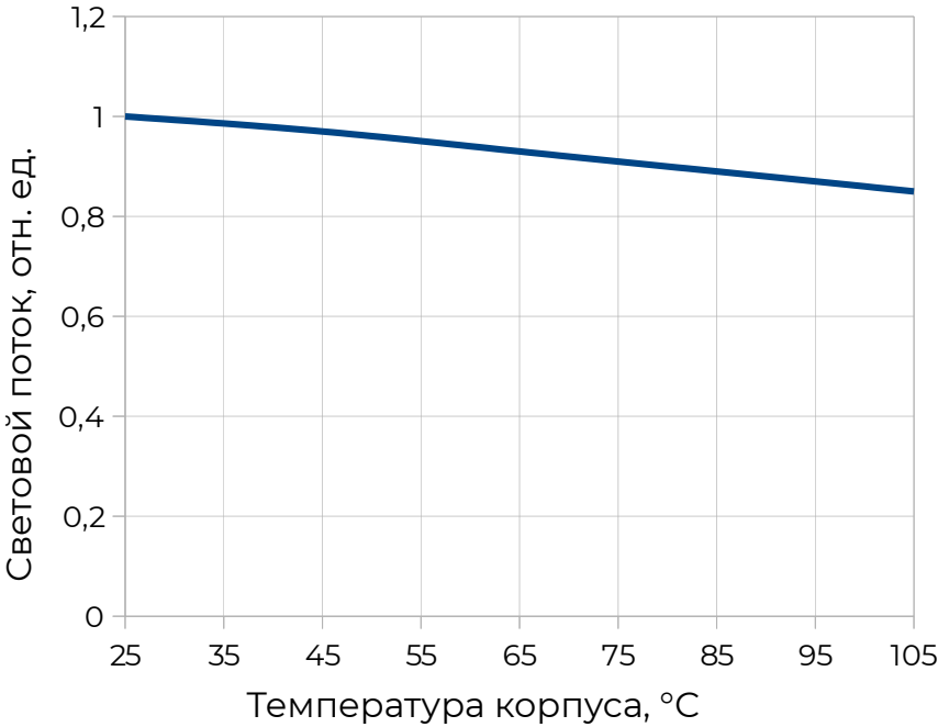
Зависимость светового потока от температуры перехода (IF = 50мА, Tj = 25 °С)
