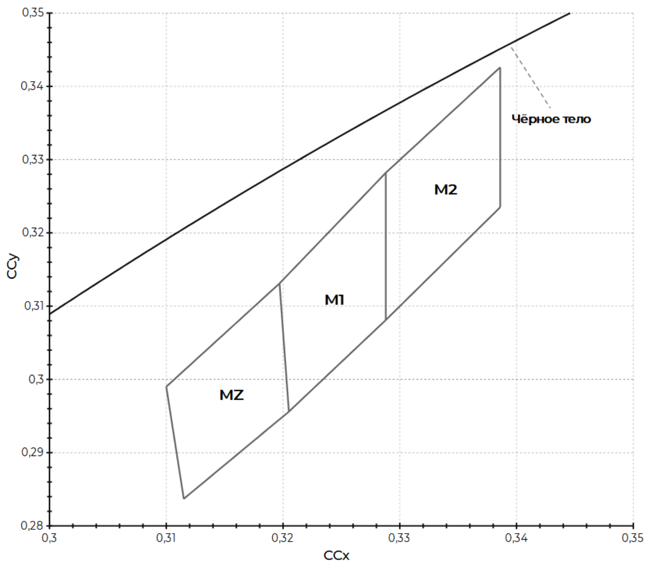
Рисунок 1. График кодов цветовых бинов (CIE 1931, IF=50 мА, TJ=25 °С)
