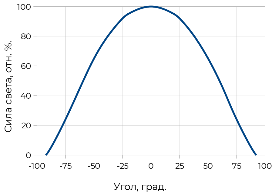
Кривая силы света (IF = 50мА, Tj = 25 °C)
