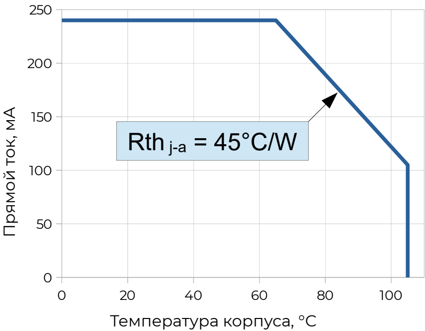
Область безопасной работы
