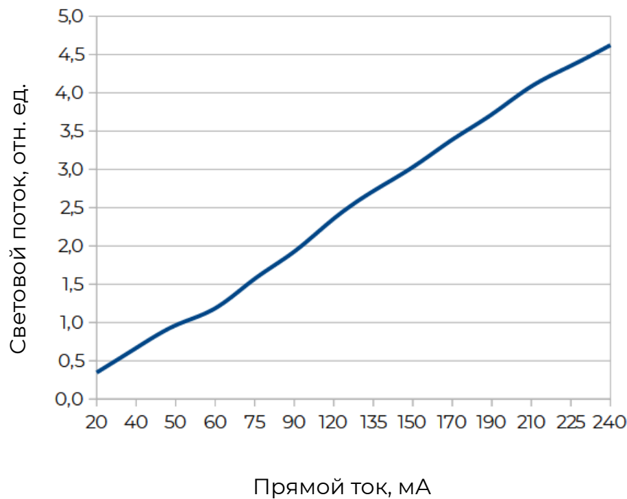
Зависимость светового потока от прямого тока (Tj = 25 °C)
